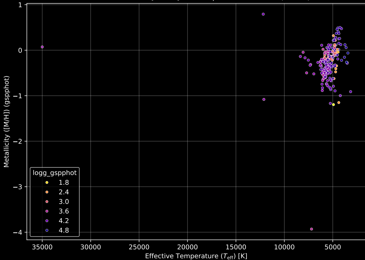
APOGEE DR17 Field: [165-30] Stellar Population Parameters (n= 215)
